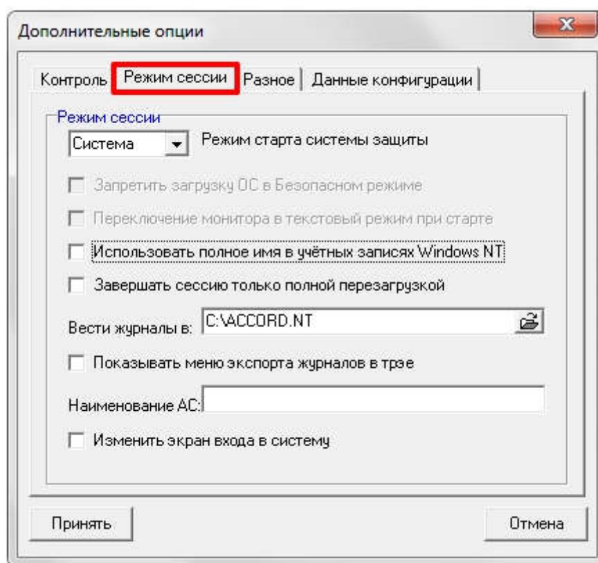
Рисунок 24 - Дополнительные параметры «Режим сессии» в настройке СЗИ
