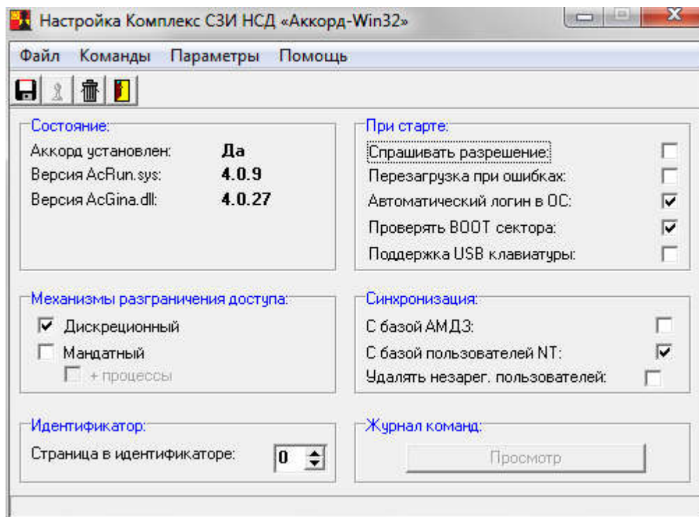
Рисунок 5 - Главное окно программы настройки комплекса «Аккорд»
